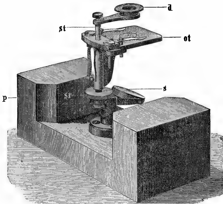
Фиг. 12. Малый препарирный микроскопъ Цейсса на препарирной ножкѣ, въ \frac{2}{3} натур. величины. ot предметный столикъ, d дублетъ, st передвижная рукоятка, st винтъ для точной установки, s зеркало, p колодки препарирной ножки
